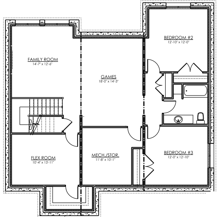
BASEMENT PLAN - 1145 SQ.FT.
