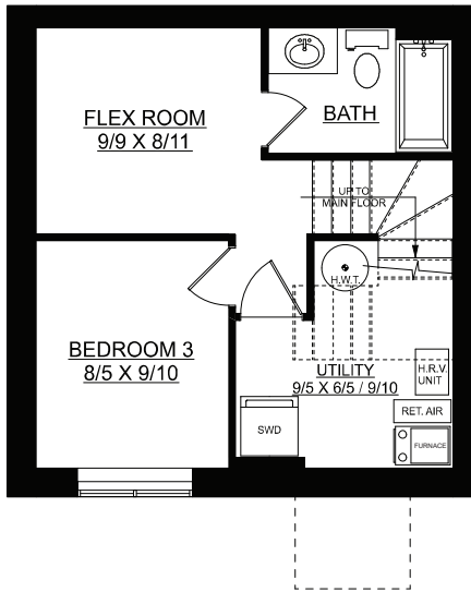
OPTIONAL BASEMENT PLAN 290 SQ.FT
